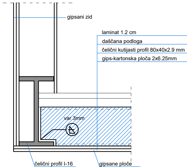
DETALJ VEZE ČELIČNIH PROFILA GALERIJE - D1
